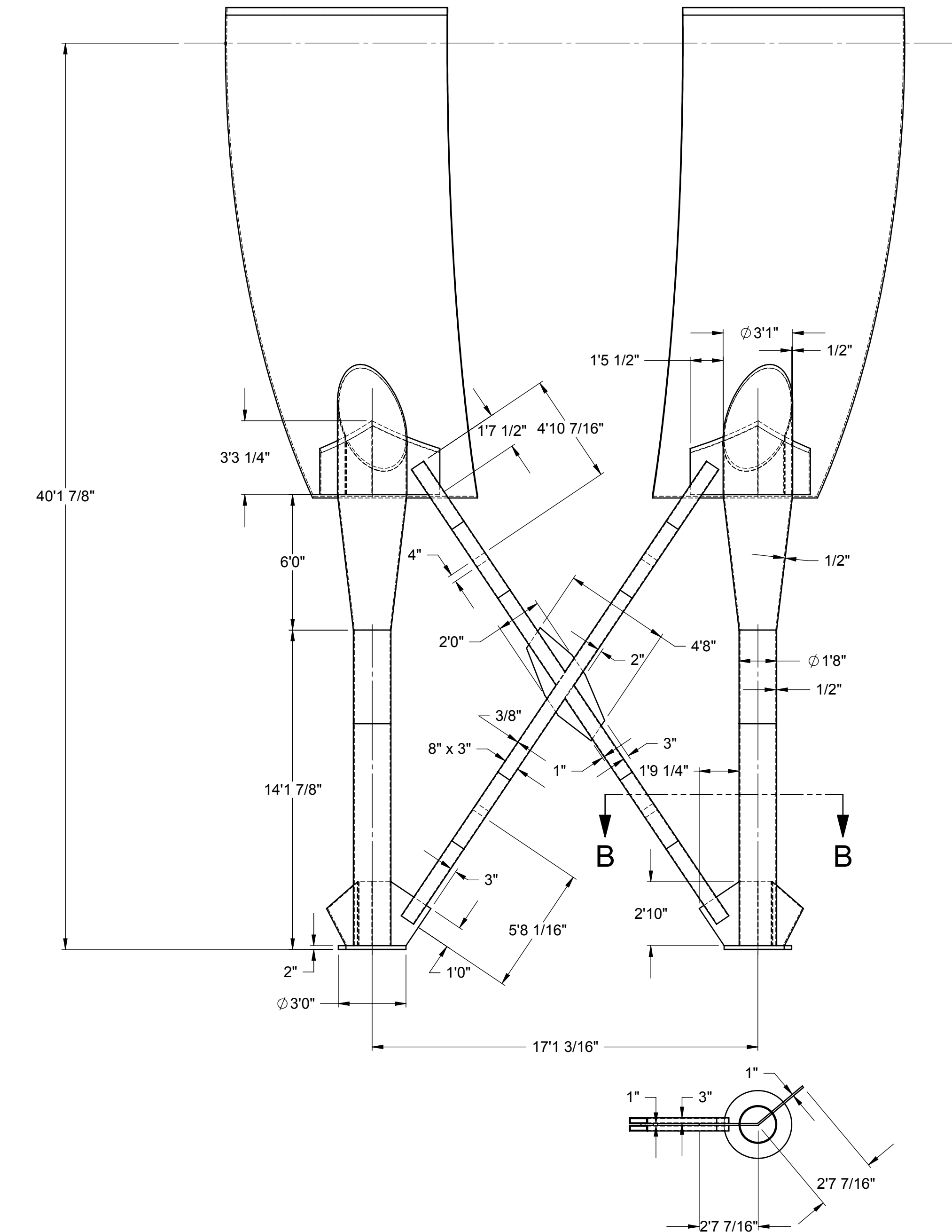
SECTION B-B SCALE 1 : 48
